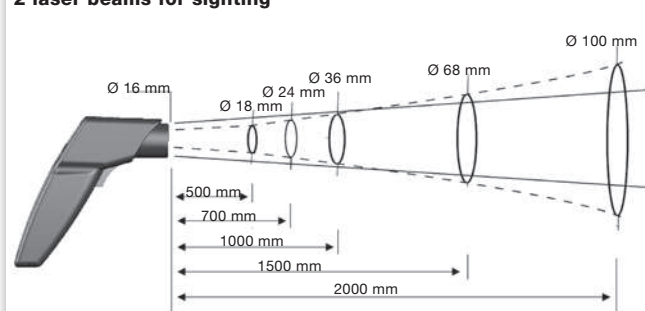
testo 830-T4
